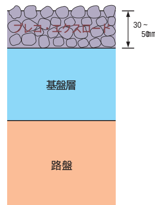
標準断面図
